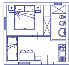
5,00 mt C1-C2 A Bilo Fig. 3
