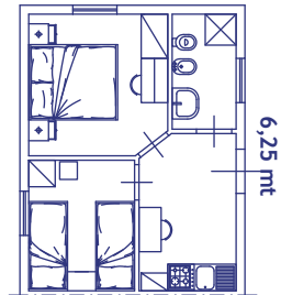
4,80 mt C3 - Trilo Fig. 5
