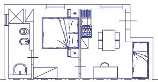
7,65 mt C2B - Bilo Fig. 4
